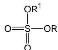
sulfato de dialquilo
