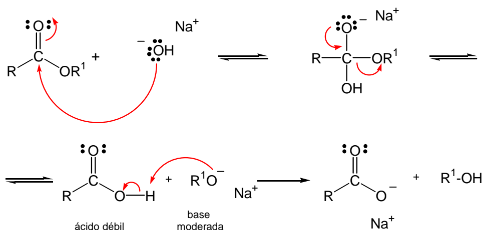
Figura 45. Mecanismo de la reacción de saponificación.
