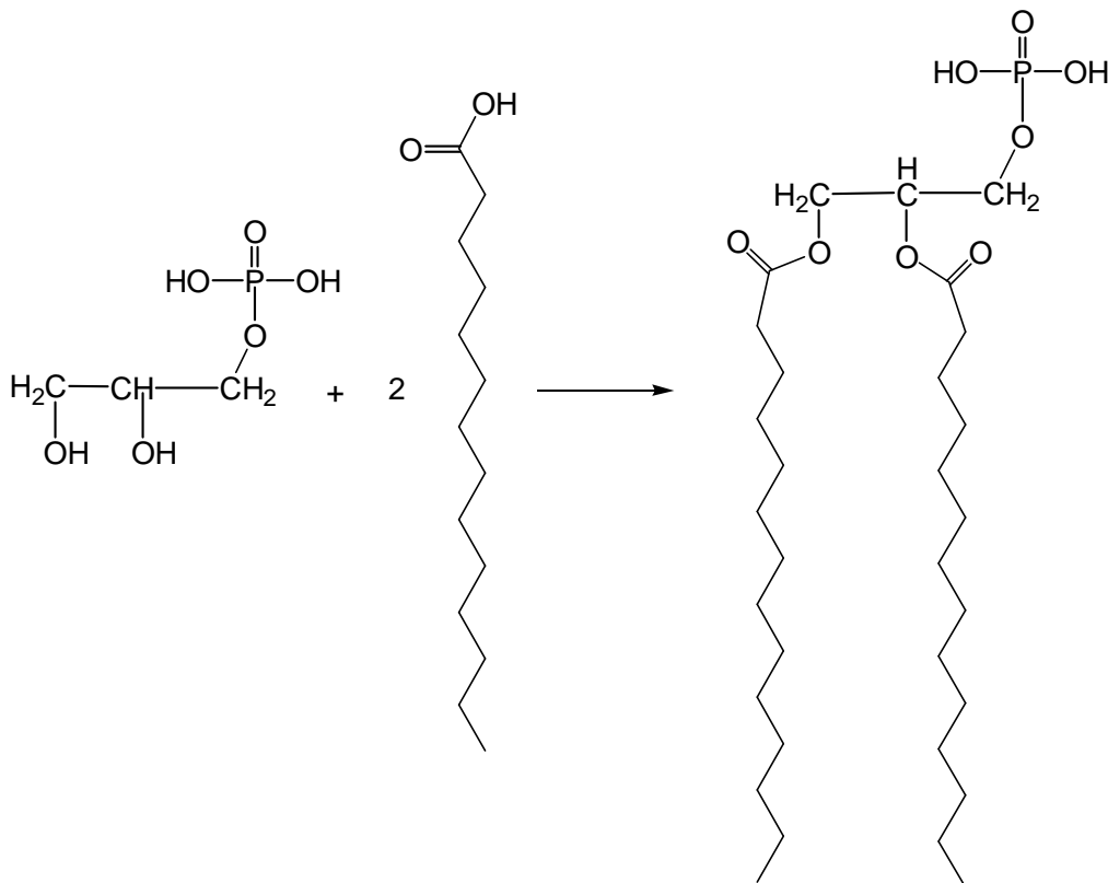
Formación de un ácido fosfatídico
